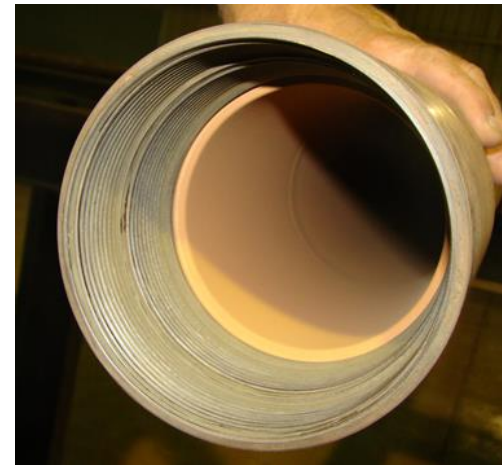
Tubería de Producción Recubierta Internamente. Fuente Ecopetrol S.A.
